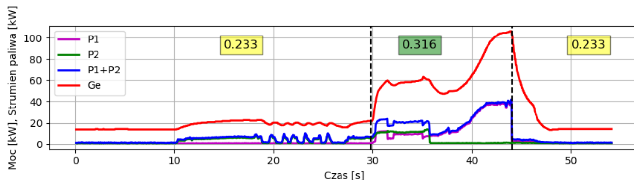
Rys. 7 Cykl nr 2. Przebieg mocy układu hydraulicznego oraz mocy paliwa oraz średnia sprawność w danej fazie cyklu
